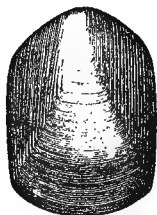
ORTHOSINA VERNEULI. LITUITES CORNU-ARIETIS. LINGULA LOWISII.
